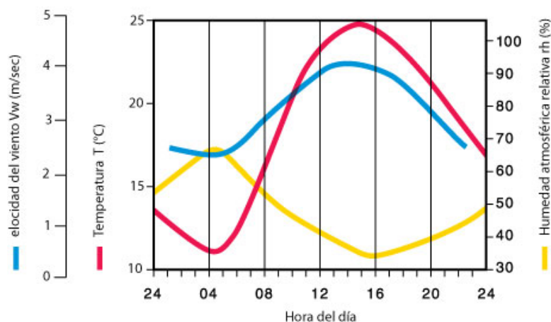
Figura 14. Evolución de la temperatura y humedad relativa a lo largo del día.
