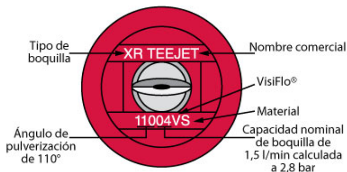
Figura 4. Características de una boquilla de abanico plano
