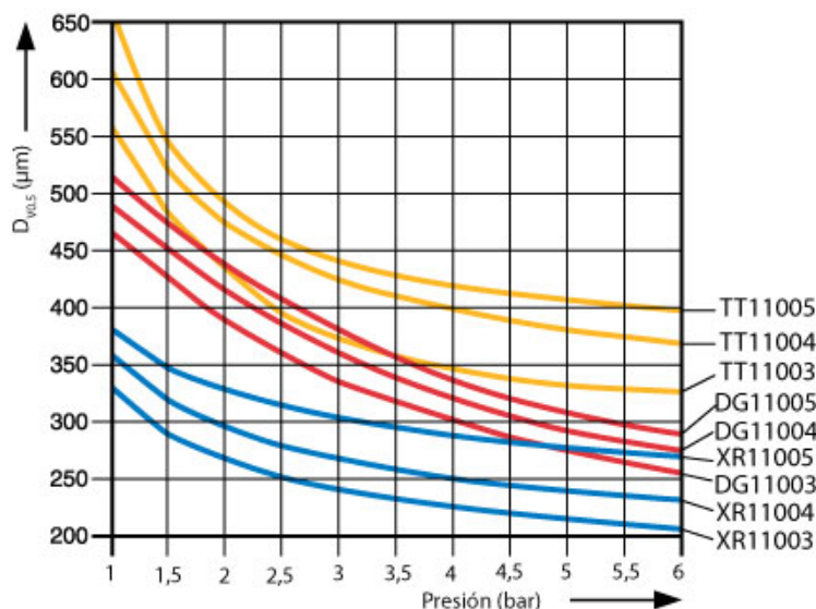
Figura 11. Diámetro de gotas de diferentes boquillas a diferentes presiones.
