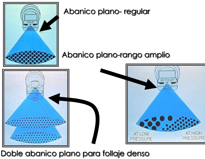
Figura 7. Características de las boquillas Spraying Systems
