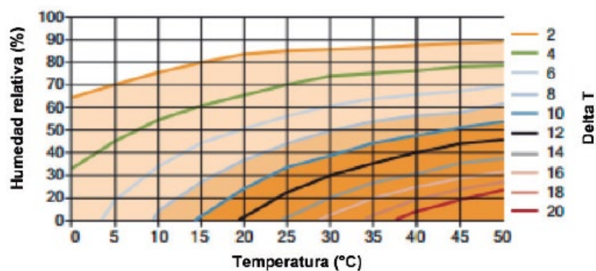
Figura 13. Valores de Delta T en función de la humedad relativa y la temperatura
