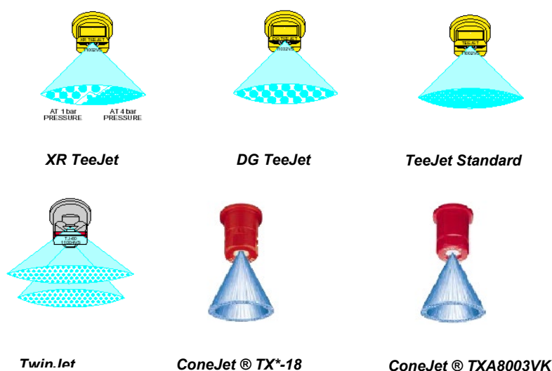
Figura 6. Características de diferentes tipos de boquillas. Spraying Systems
